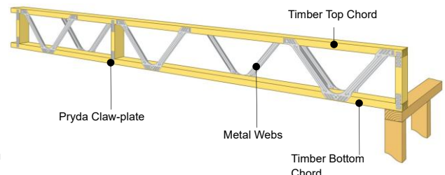
SPACEJOIST™ TRUSS
